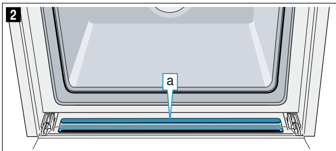
盛水盘 a 位于烹饪箱下 (图 2)。
